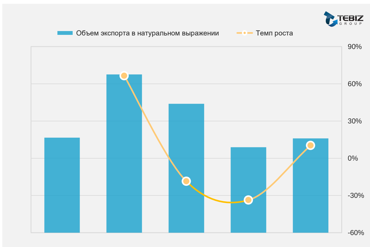
График. Динамика казахстанского экспорта электродов для сварки в натуральном выражении в 2021-2025 гг.
