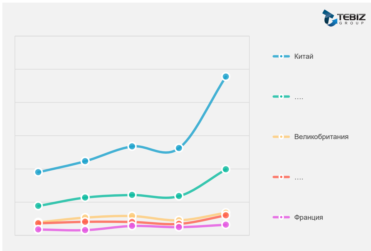
Диаграмма. Структура казахстанского импорта кранов по крупнейшим странам в натуральном выражении в 2021-2025 гг.
