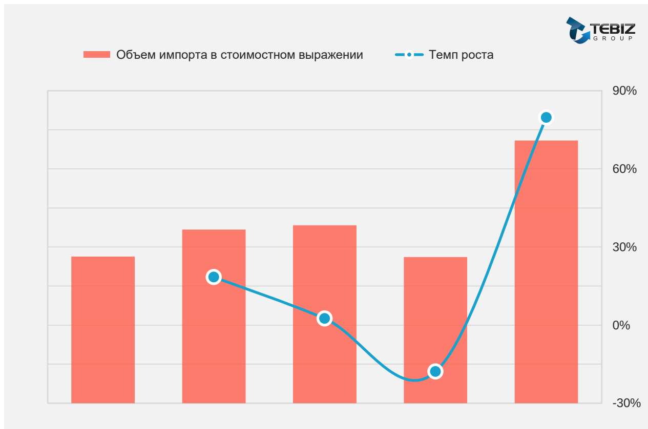
График. Динамика казахстанского импорта кранов в стоимостном выражении 2021-2025 гг., [тыс.долл]
