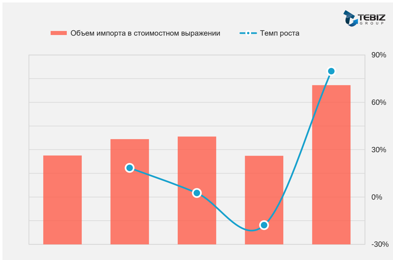
График. Динамика казахстанского импорта кварца в стоимостном выражении 2021-2025 гг., [тыс.долл]
