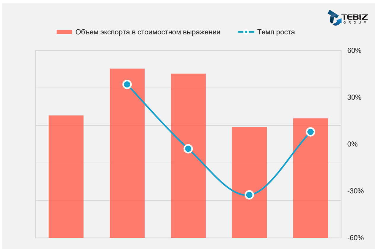
График. Динамика казахстанского экспорта кварца в стоимостном выражении 2021-2025 гг., [тыс.долл]
