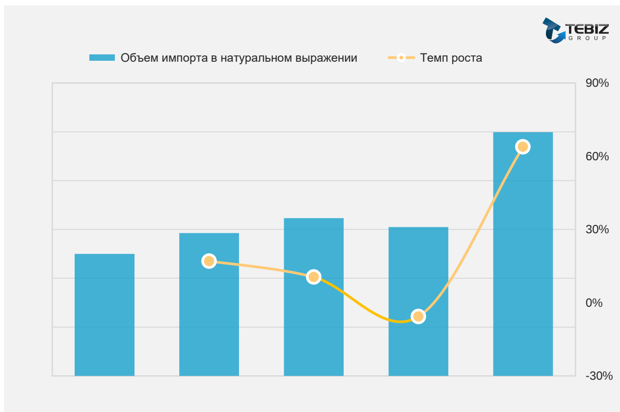
График. Динамика казахстанского импорта лома цветных металлов в натуральном выражении в 2021-2025 гг.
