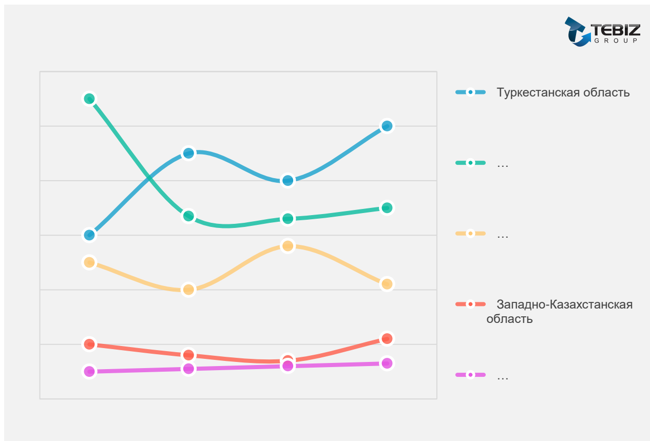
График. Структура казахстанского экспорта лома цветных металлов по основным областям в натуральном выражении в 2021-2025 гг.
