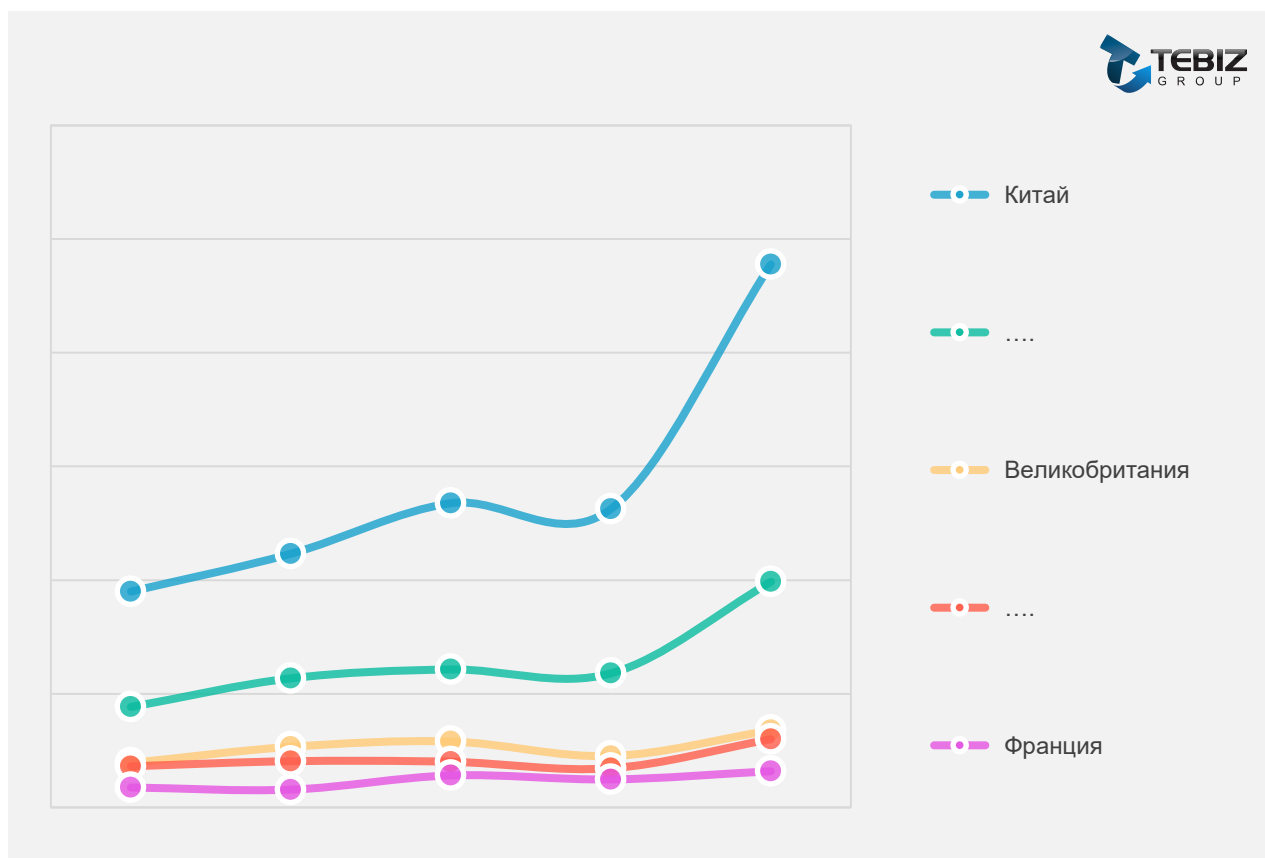
Диаграмма. Структура казахстанского импорта металлического крепежа по крупнейшим странам в натуральном выражении в 2021-2025 гг.
