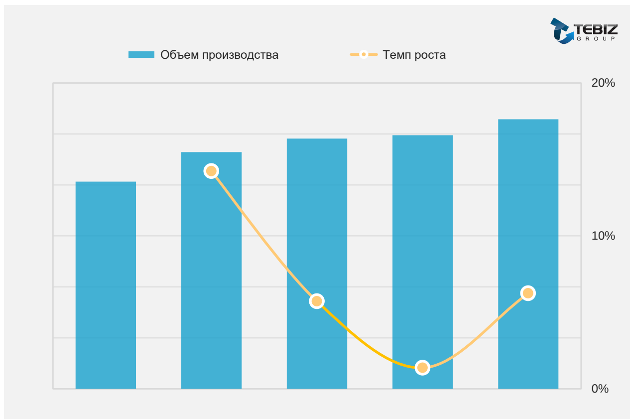
График. Динамика объемов производства оборудования для фильтрации жидкостей в Казахстане в 2021-2025 гг.
