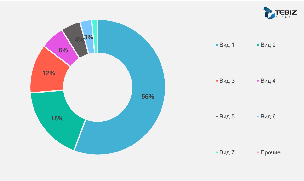
Диаграмма. Сегментация казахстанского рынка оборудования для фильтрации жидкостей по видам в ... г., [%]
