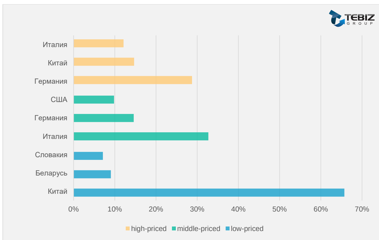
Диаграмма. Лидирующие страны по импорту балансировочных станков в Россию по ценовым сегментам в натуральном выражении, [%]
