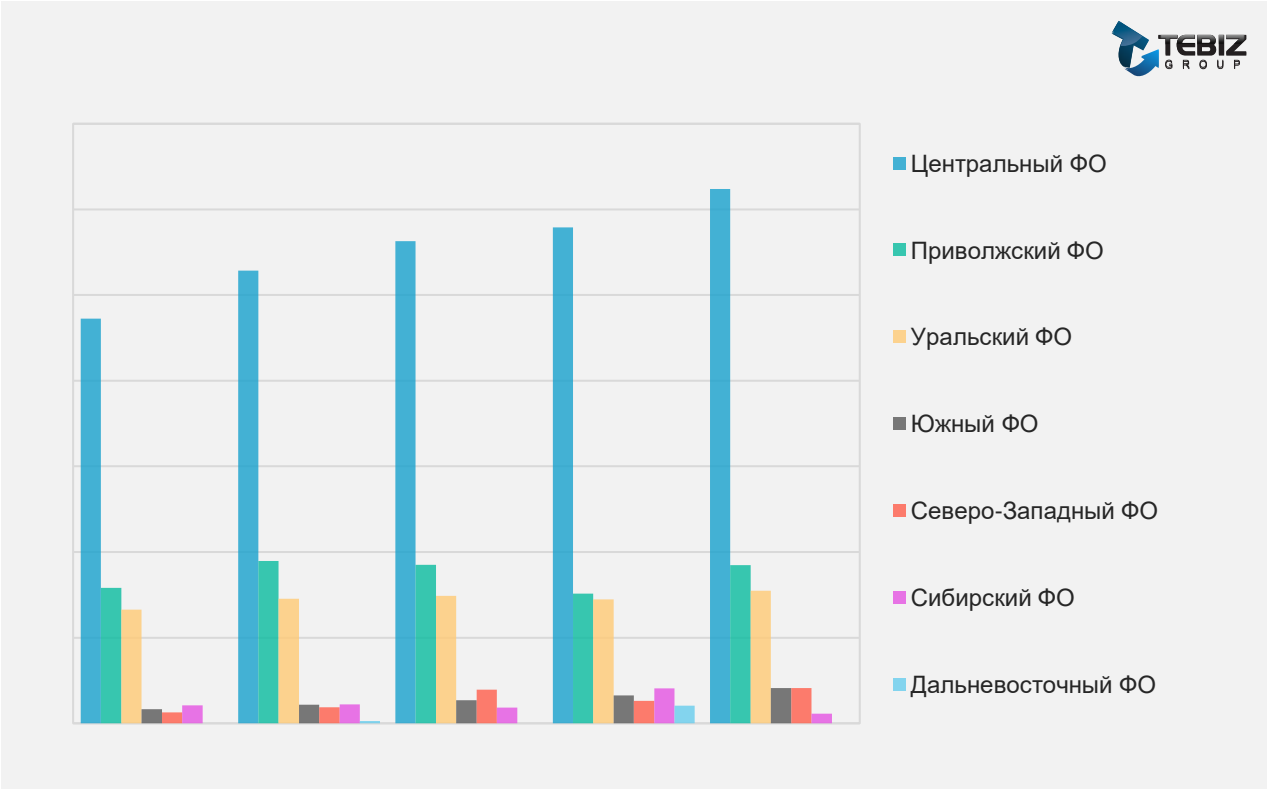
Диаграмма. Динамика производства металлургических конвертеров по федеральным округам России в 2021-2025 гг.
