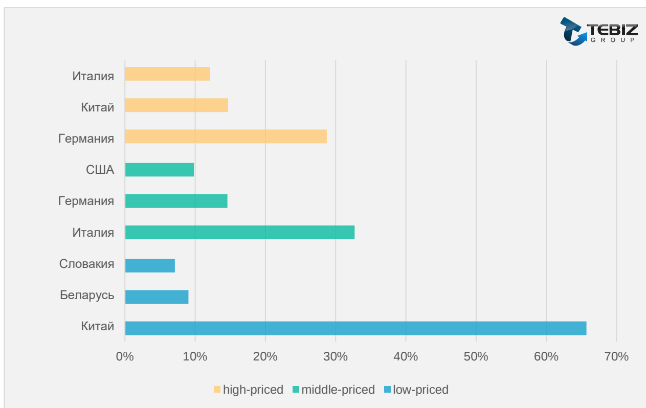
Диаграмма. Лидирующие страны по импорту прессматериала SMC в Россию по ценовым сегментам в натуральном выражении, [%]
