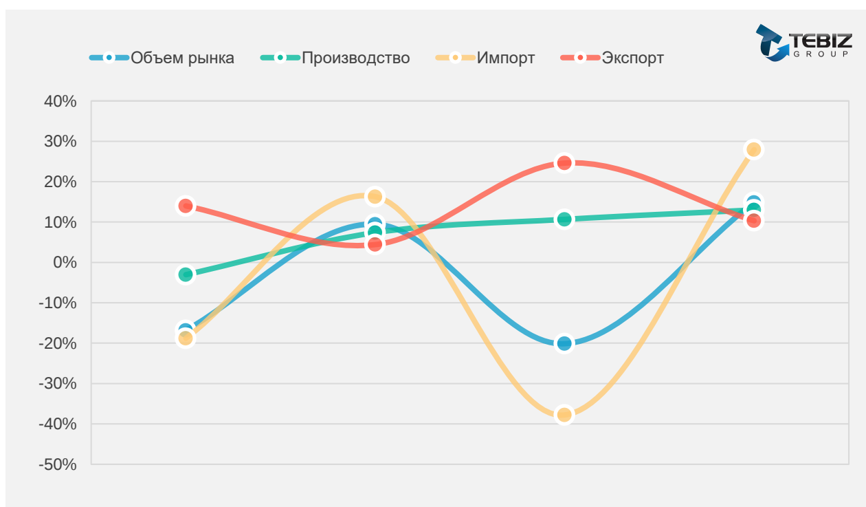
График. Темпы роста основных показателей рынка шин для строительной техники
