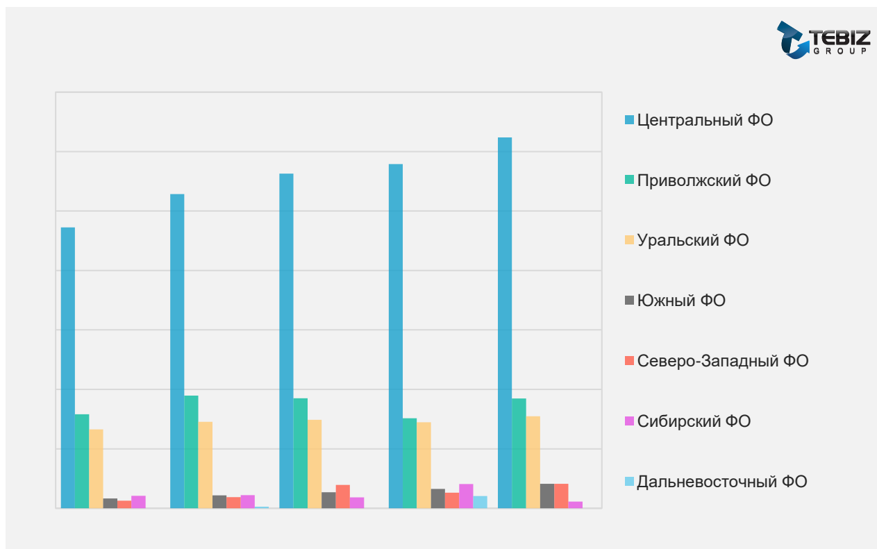
Диаграмма. Динамика производства стальных строительных конструкций по федеральным округам России в 2021-2025 гг.
