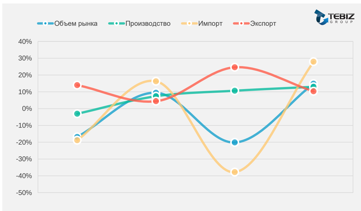
График. Темпы роста основных показателей рынка стеклопластиковой арматуры
