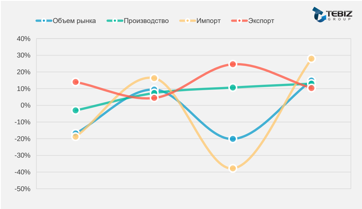
График. Темпы роста основных показателей рынка токарно-винторезных станков
