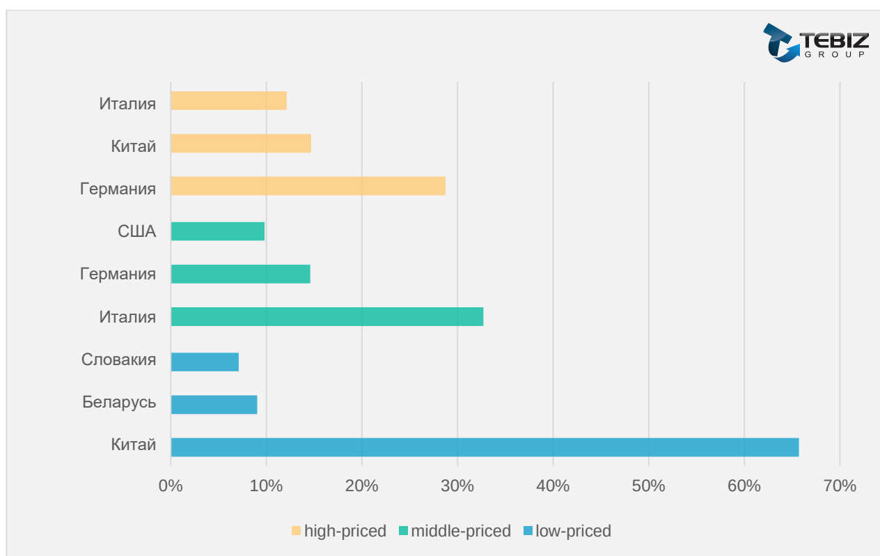
Диаграмма. Лидирующие страны по импорту уровнемеров для сыпучих материалов в Россию по ценовым сегментам в натуральном выражении, [%]
