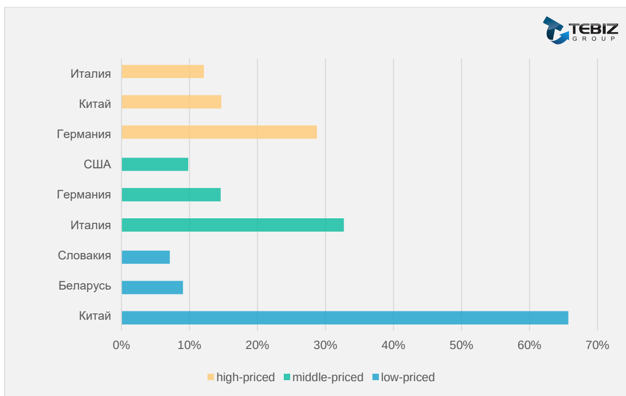
Диаграмма. Лидирующие страны по импорту железнодорожных подвижных составов в Россию по ценовым сегментам в натуральном выражении, [%]
